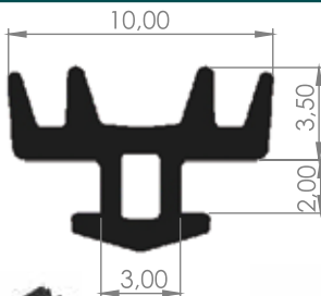
ALM. LEKSAN FİTİL 09-38
