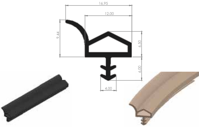
09 - 08 AHŞAP KAPI FİTİLİ
