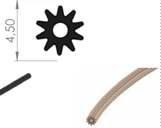
114,5-SİNEKLİK FİTİLİ 4,5MM
