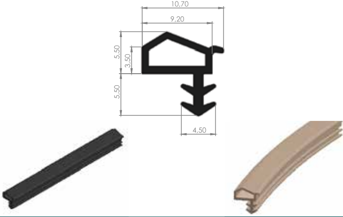
09 - 32 AHŞAP KAPI FİTİLİ
