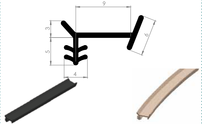
09 - 25 AHŞAP KAPI FİTİLİ
