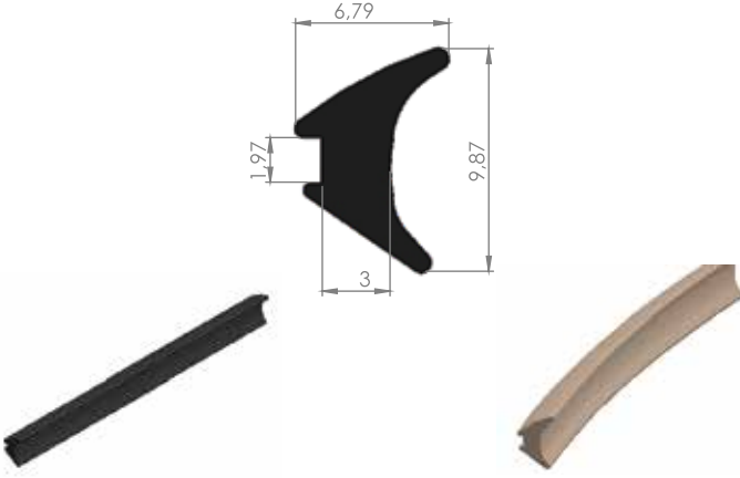
ALÜMİNYUM 05-07 3MM KAMA
