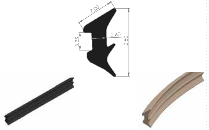
05-16 2.60MM TIRNAKLI KAMA
