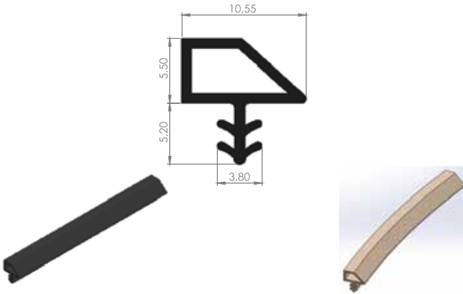
09 - 11 AHŞAP KAPI FİTİLİ
