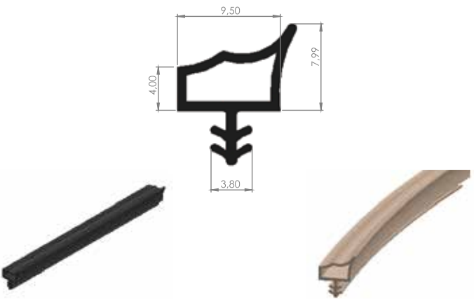
09 - 30 AHŞAP KAPI FİTİLİ
