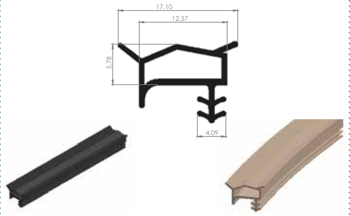
09 - 29 AHŞAP KAPI FİTİLİ
