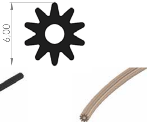
116-SİNEKLİK FİTİLİ 6MM
