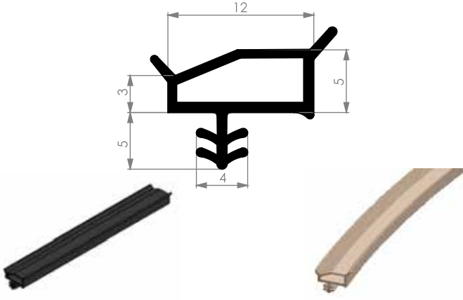
KOMPOZİT KASA FİTİLİ 10-02
