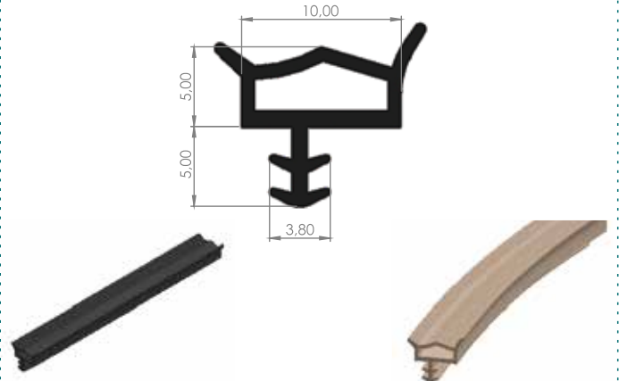
09-34 AHŞAP KAPI FİTİLİ
