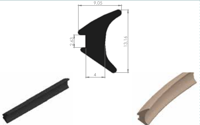
ALÜMİNYUM 05-08 4MM KAMA
