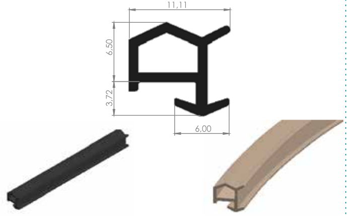
KOMPOZİT KASA FİTİLİ 10-01
