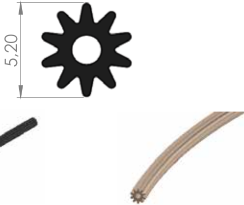
115,2-SİNEKLİK FİTİLİ 5,2MM
