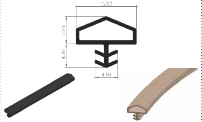
09 - 07 AHŞAP KAPI FİTİLİ-12mm
