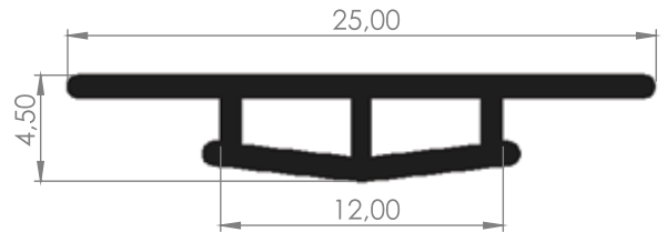
152-008 SNK KAPAMA FİTİLİ
