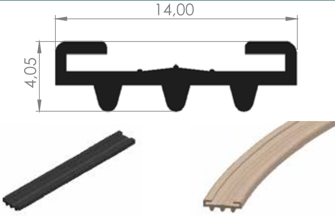
KELEPÇE FİTİLİ 12LİK
