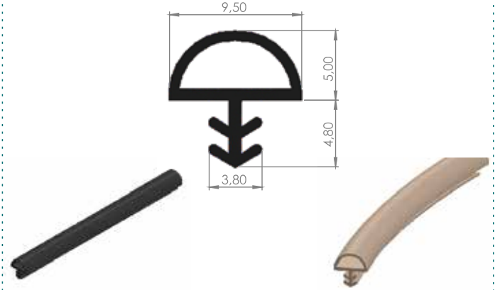
09 - 10 AHŞAP KAPI FİTİLİ
