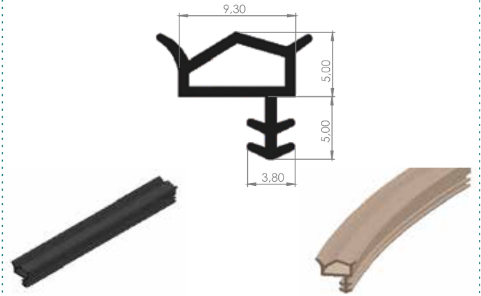
09 - 16 AHŞAP KAPI FİTİLİ
