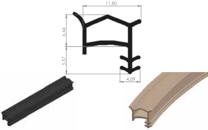
09 - 01 AHŞAP KAPI FİTİLİ
