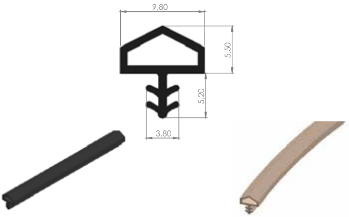
AHŞAP KOD 09-07 10mm
