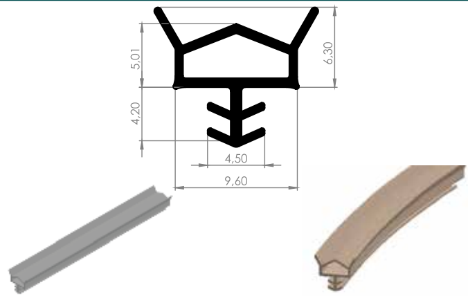
09 - 17 AHŞAP KAPI FİTİLİ
