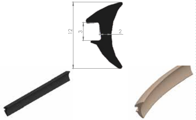
ALÜMİNYUM 05-06 2MM KAMA
