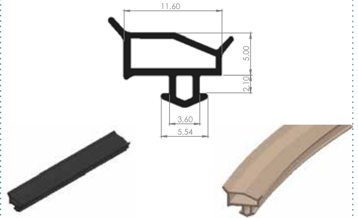
KOMPOZİT KASA FİTİLİ 10-03
