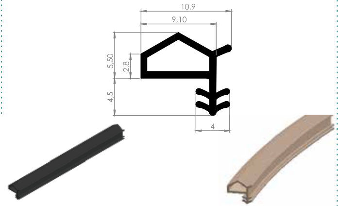
09 - 06 AHŞAP KAPI FİTİLİ
