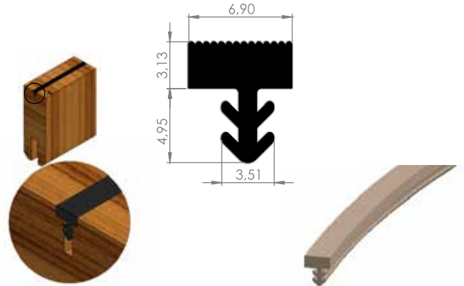
09 - 35 AHŞAP KAPI FİTİLİ
