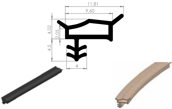
09 - 28 AHŞAP KAPI FİTİLİ
