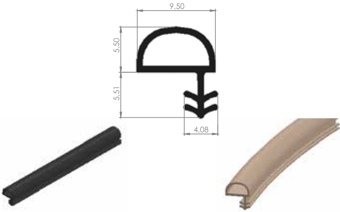
09 - 05 AHŞAP KAPI FİTİLİ
