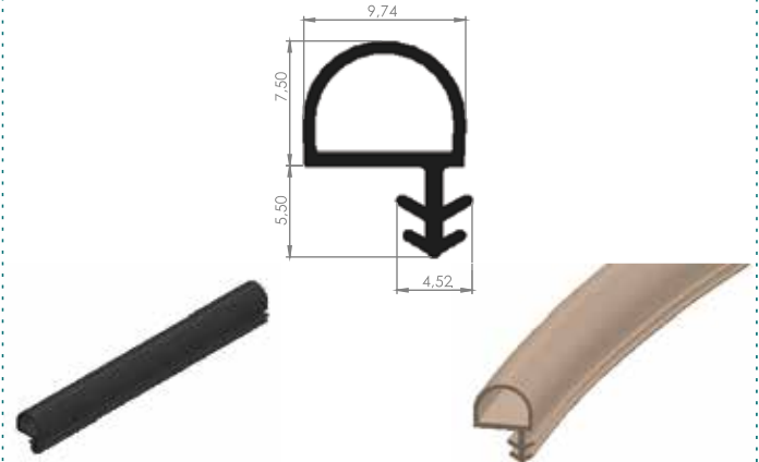
09 - 02 AHŞAP KAPI FİTİLİ
